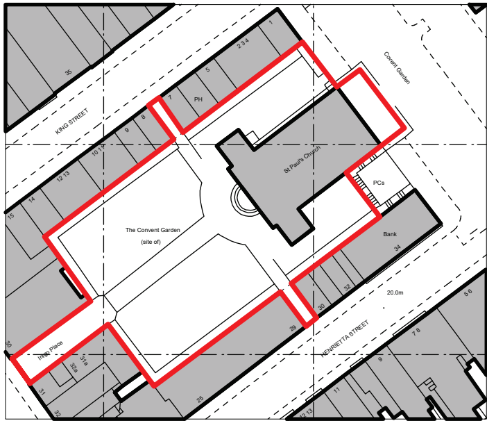
1:1250 Site Plan
