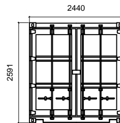
Door Elevation
