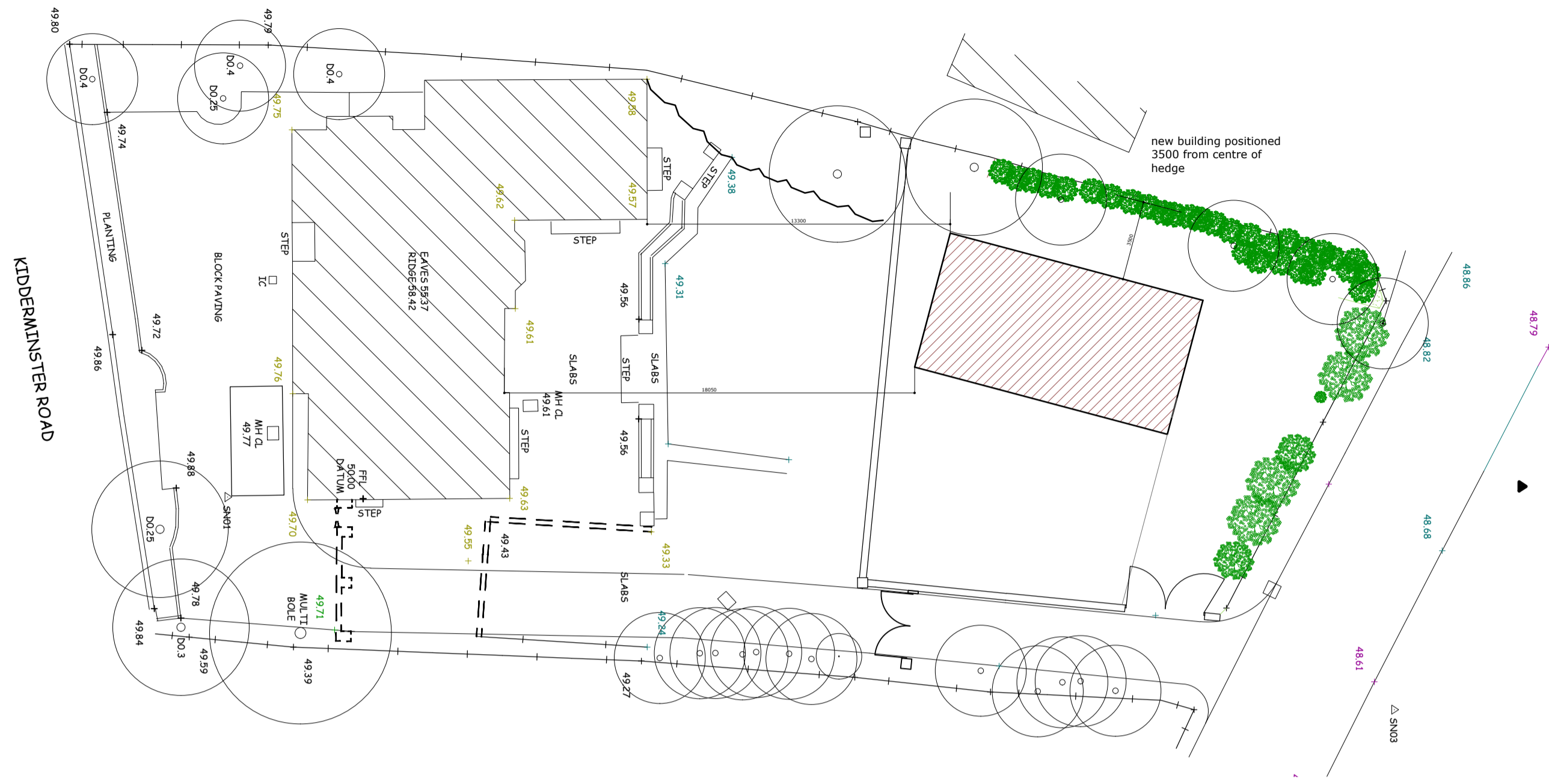
Site Plan 1:200
