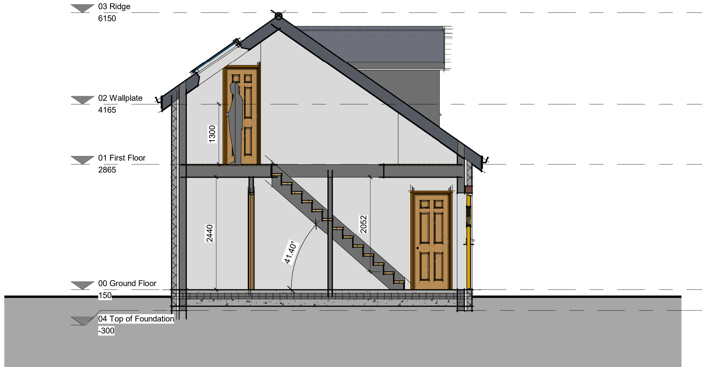
1 Section 1 1 : 50
