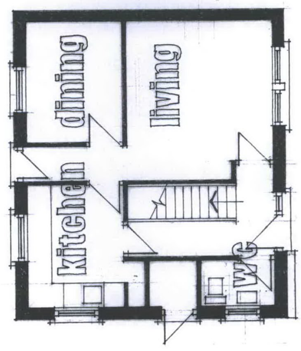
G-F plan
