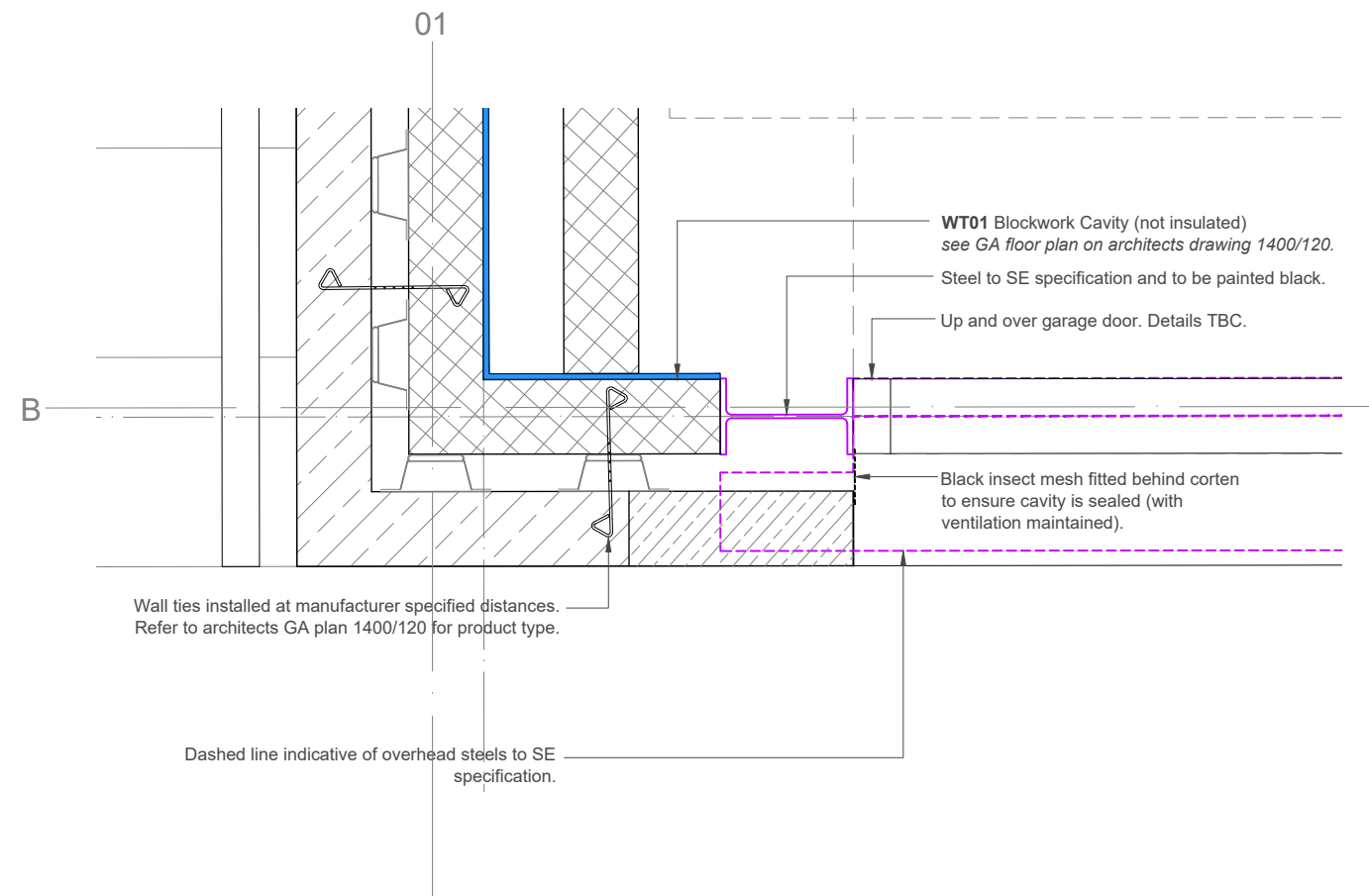
02 - D0.01/01 Jamb Detail
