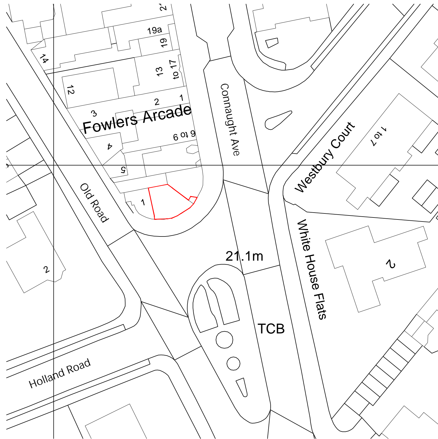
Site Plan 1:500
