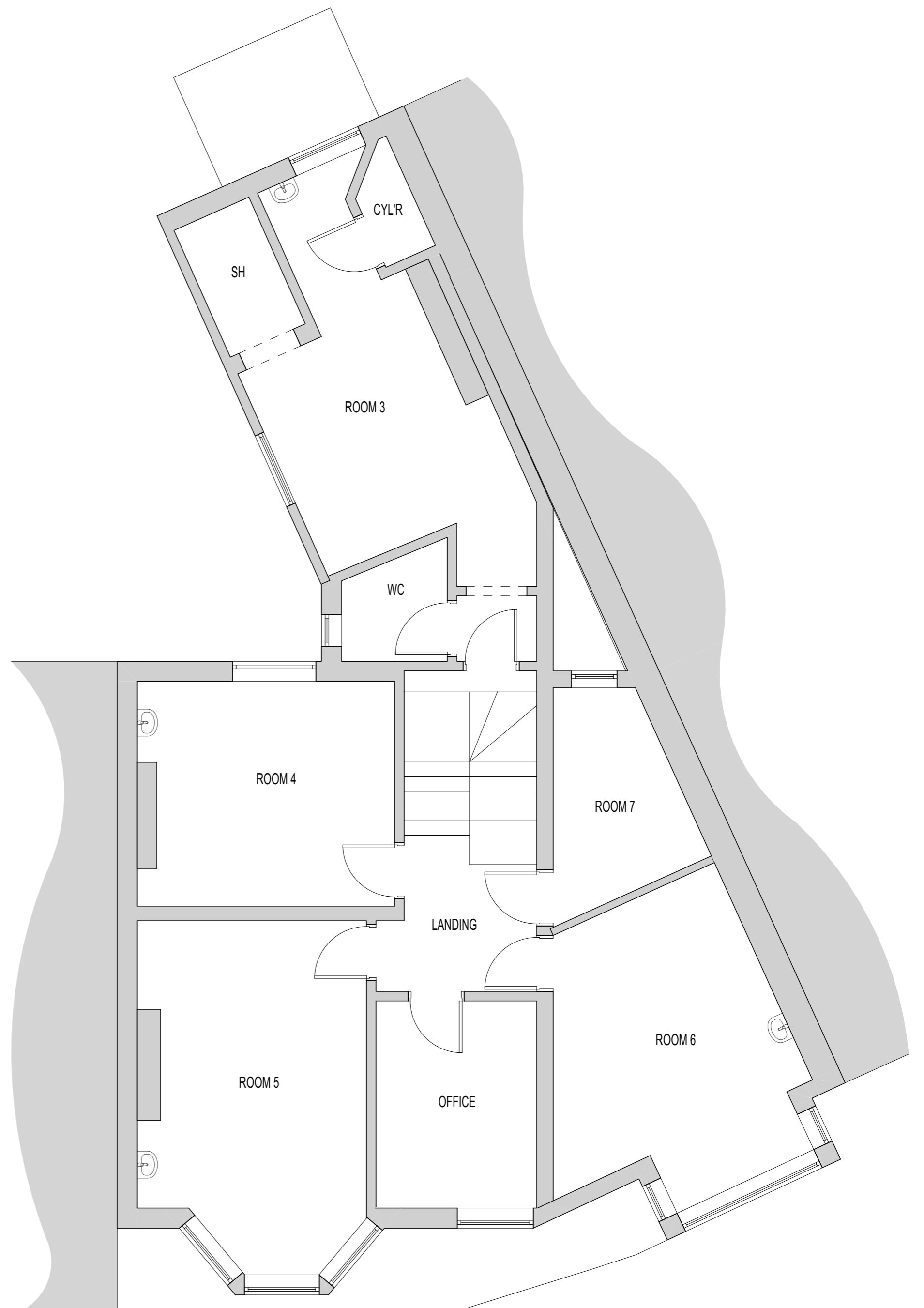
Existing FF Layout Scale: 1:50
