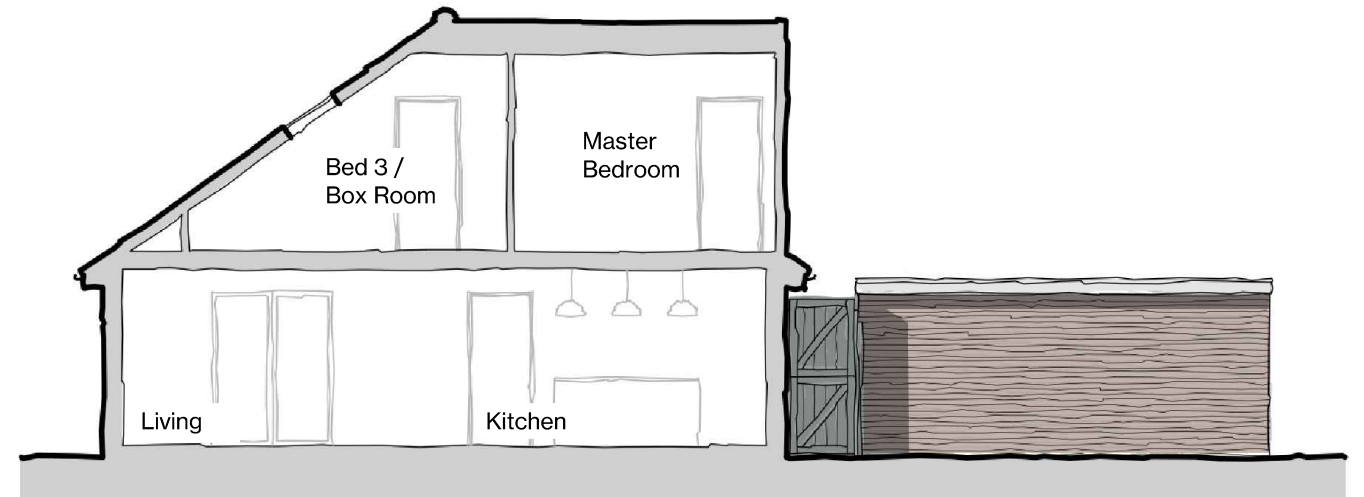
Side SE Elevation 1:100
