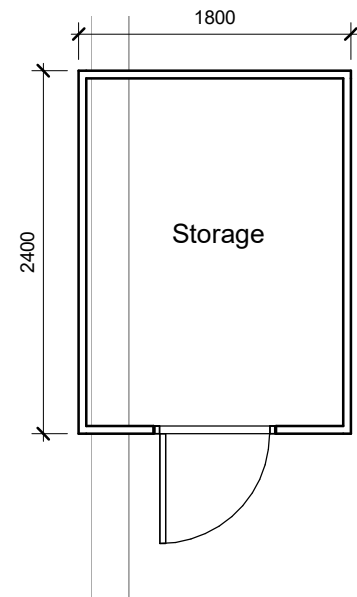
Floor Plan 1 : 50
